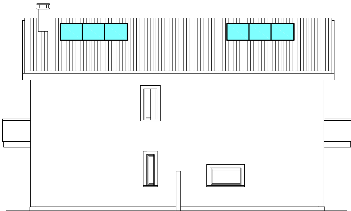
Prospetto Ovest
