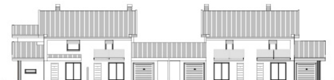
PROSPETTO SUD
