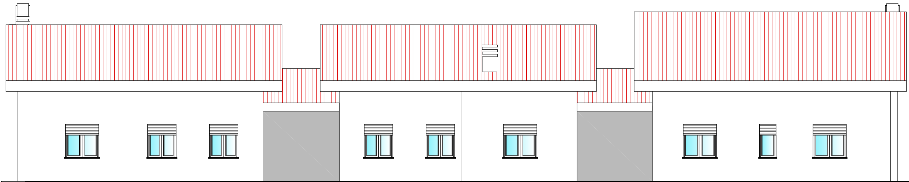
PROSPETTO OVEST
