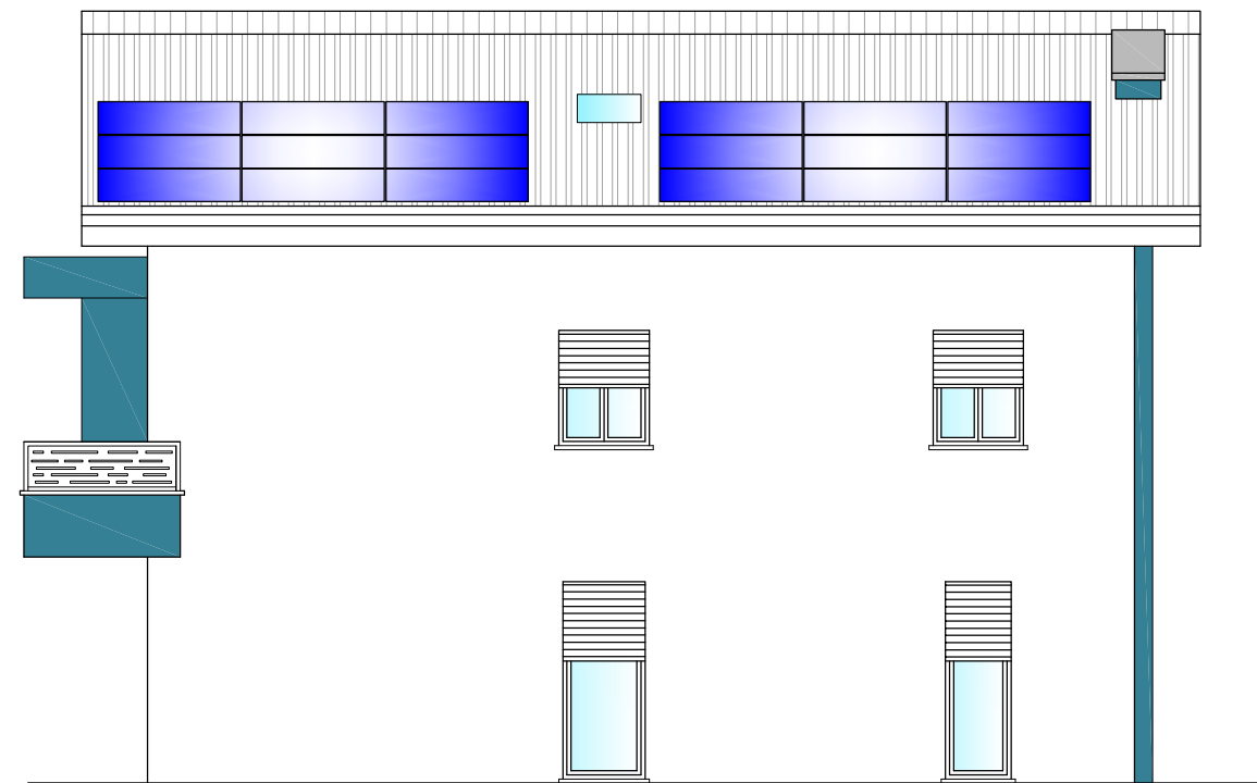
PROSPETTO SUD
