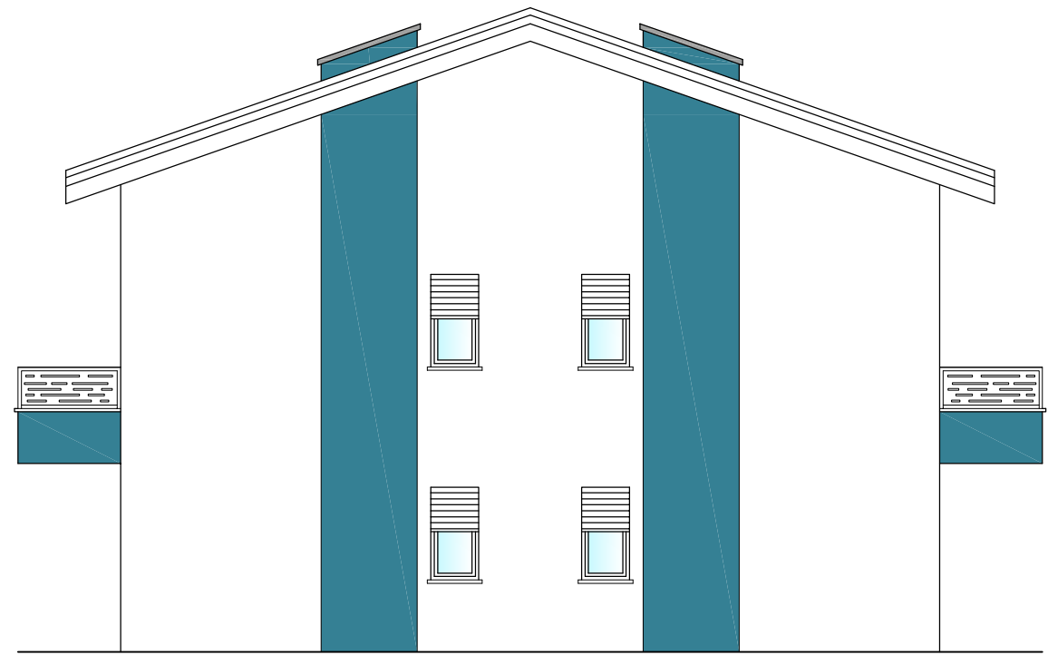
PROSPETTO EST
